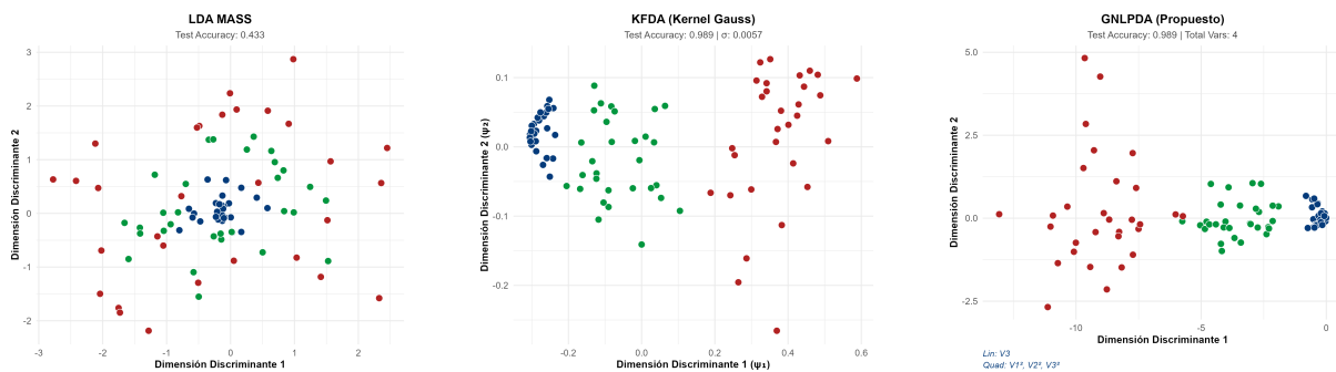
Figura 5.10: Comparativa geométrica de los espacios de proyección para el conjunto de datos cebolla 3D.
