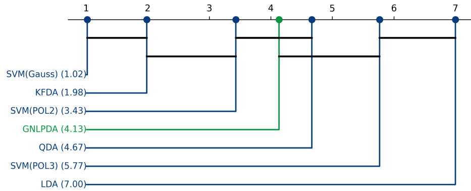
Figura 5.37: Análisis de significancia estadística post-hoc mediante distancias críticas de Nemenyi para el conjunto de datos cebolla 20D.
