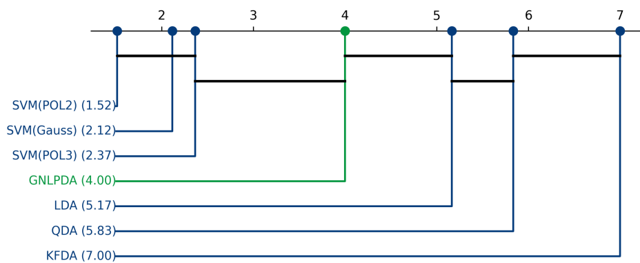
Figura 5.43: Análisis de significancia estadística post-hoc mediante distancias críticas de Nemenyi para el conjunto de datos Indicadores 2015.
