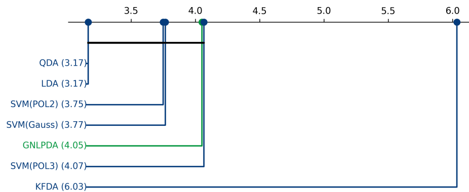
Figura 5.19: Análisis de significancia estadística post-hoc mediante distancias críticas de Nemenyi para el conjunto de datos Palmer penguins.
