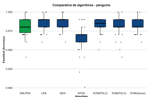
Figura 5.18: Distribución empírica del rendimiento predictivo para el conjunto de datos Penguins.
