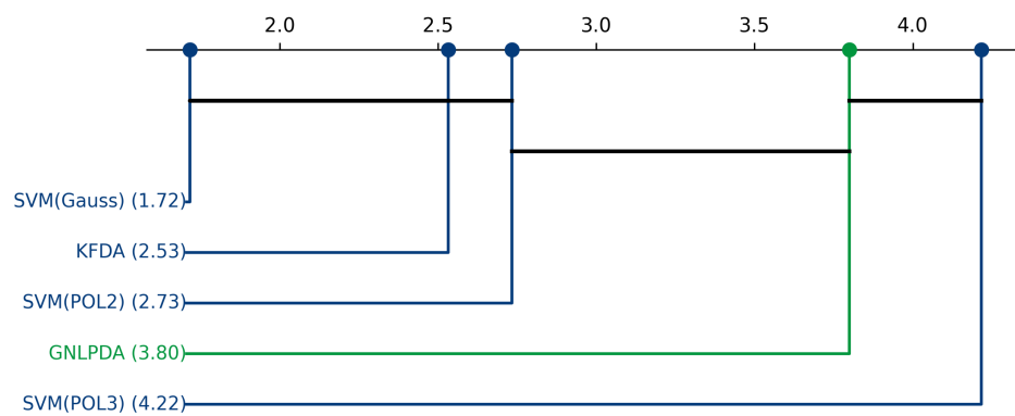
Figura 5.29: Análisis de significancia estadística post-hoc y corrección por enmascaramiento mediante distancias críticas de Nemenyi para el conjunto de datos Ionosphere.
