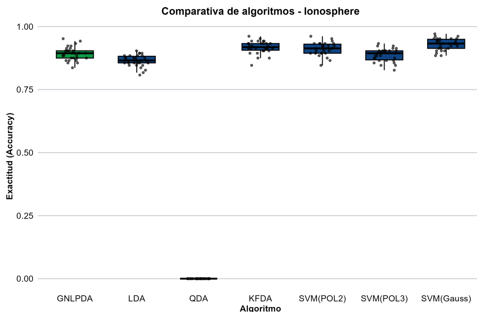
Figura 5.27: Distribución empírica del rendimiento predictivo para el conjunto de datos Ionosphere.
