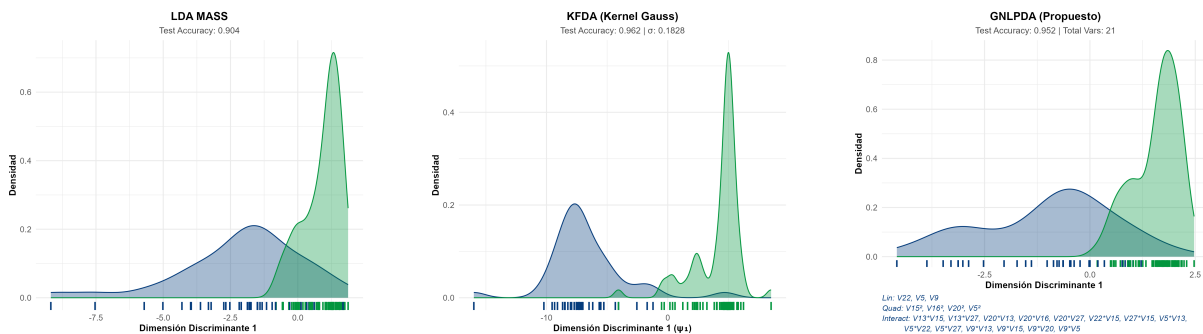
Figura 5.9: Comparativa geométrica de los espacios de proyección para el conjunto de datos Ionosphere.
