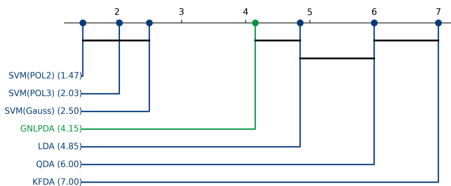
Figura 5.46: Análisis de significancia estadística post-hoc mediante distancias críticas de Nemenyi para el conjunto de datos Indicadores 2020.
