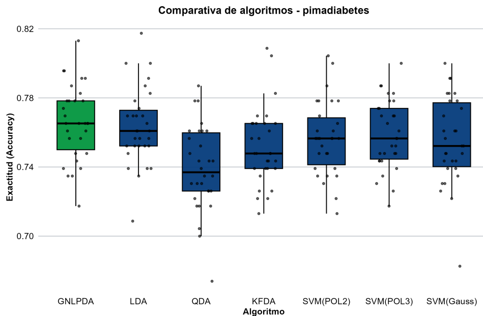
Figura 5.39: Distribución empírica del rendimiento predictivo para el conjunto de datos Pima diabetes.
