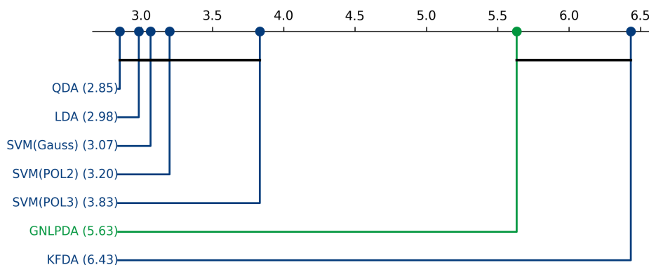
Figura 5.22: Análisis de significancia estadística post-hoc mediante distancias críticas de Nemenyi para el conjunto de datos Wines.
