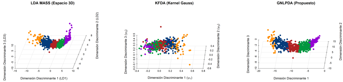
Figura 5.15: Comparativa geométrica de los espacios de proyección para el conjunto de datos Indicadores 2015 (3D).
