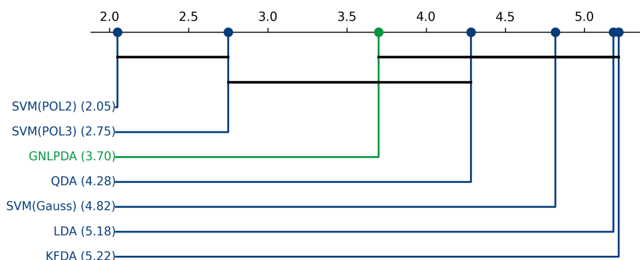
Figura 5.25: Análisis de significancia estadística post-hoc mediante distancias críticas de Nemenyi para el conjunto de datos Cancer Wisconsin.
