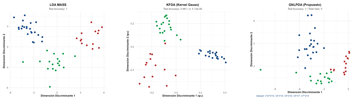
Figura 5.7: Comparativa geométrica de los espacios de proyección para el conjunto de datos Wines.
