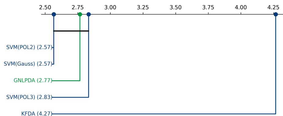
Figura 5.20: Análisis de significancia estadística post-hoc y corrección por enmascaramiento mediante distancias críticas de Nemenyi para el conjunto de datos Palmer penguins.
