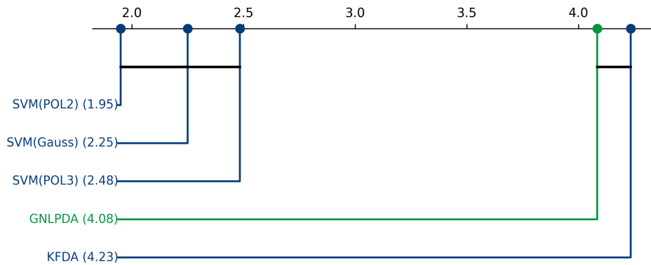
Figura 5.32: Análisis de significancia estadística post-hoc y corrección por enmascaramiento mediante distancias críticas de Nemenyi para el conjunto de datos Cebolla 3D.
