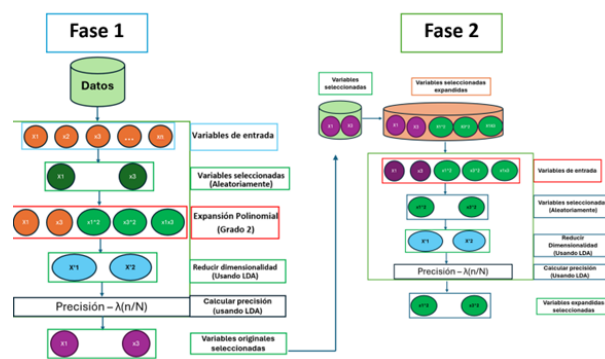
Figura 4.3: Arquitectura completa de GNLPPDA. Fuente: Elaboración propia.
