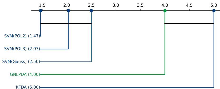
Figura 5.47: Análisis de significancia estadística post-hoc y corrección por enmascaramiento mediante distancias críticas de Nemenyi para el conjunto de datos Indicadores 2020.
