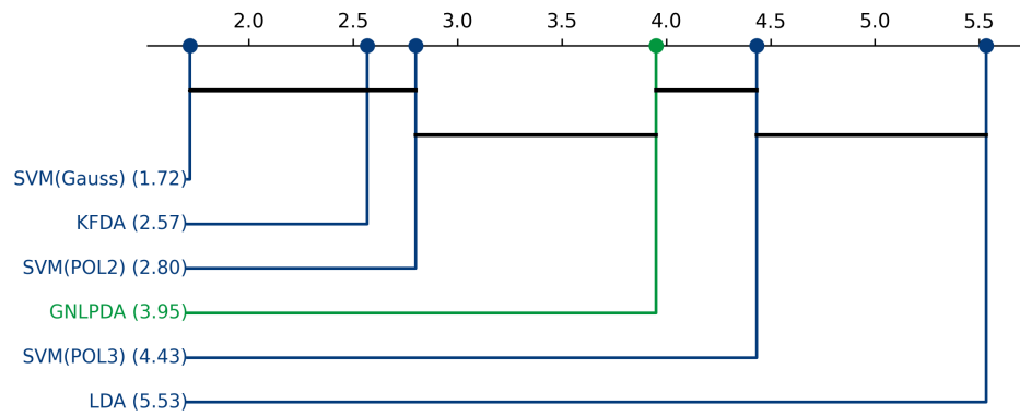
Figura 5.28: Análisis de significancia estadística post-hoc mediante distancias críticas de Nemenyi para el conjunto de datos Ionosphere.
