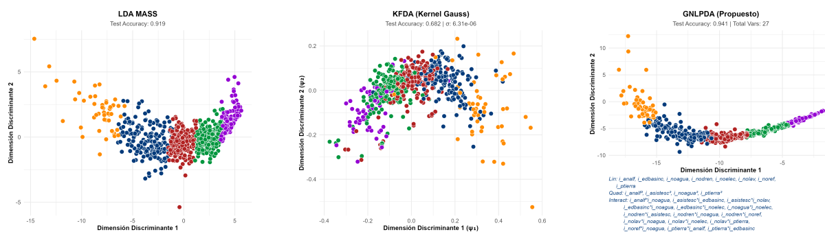
Figura 5.14: Comparativa geométrica de los espacios de proyección para el conjunto de datos Indicadores 2015 (2D).
