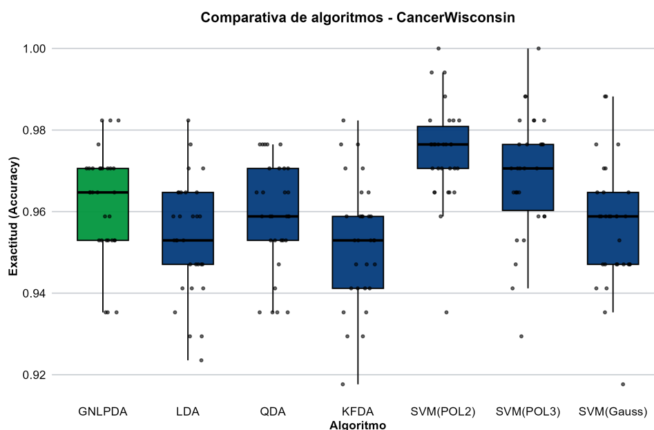
Figura 5.24: Distribución empírica del rendimiento predictivo para el conjunto de datos Cancer Wisconsin.
