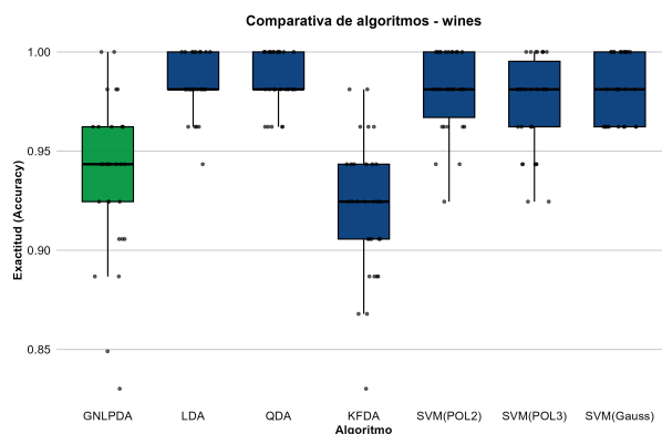
Figura 5.21: Distribución empírica del rendimiento predictivo para el conjunto de datos Wines.
