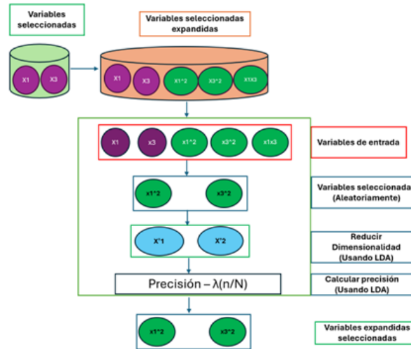
Figura 4.2: Fase II de GNLPDA: selección evolutiva de términos polinomiales sobre el espacio expandido restringido. Fuente: Elaboración propia.
