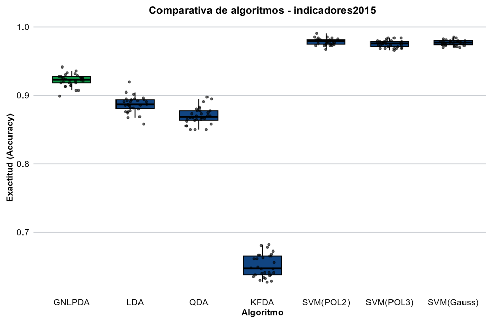
Figura 5.42: Distribución empírica del rendimiento predictivo para el conjunto de datos Indicadores 2015.
