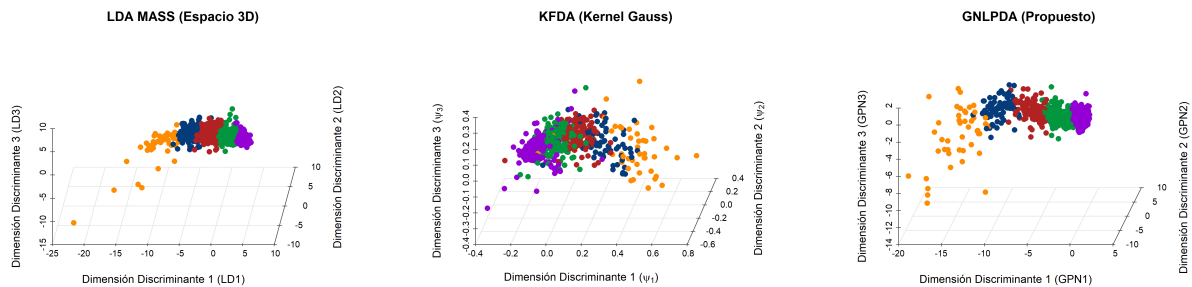
Figura 5.17: Comparativa geométrica de los espacios de proyección para el conjunto de datos Indicadores 2020 (3D).
