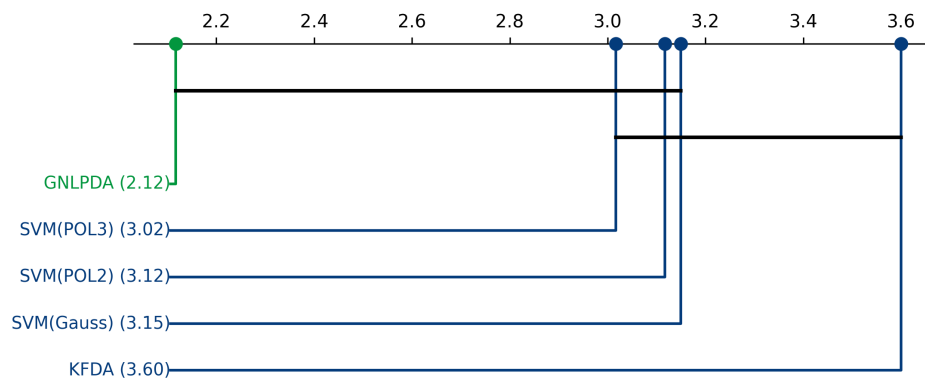
Figura 5.41: Análisis de significancia estadística post-hoc y corrección por enmascaramiento mediante distancias críticas de Nemenyi para el conjunto de datos Pima diabetes.
