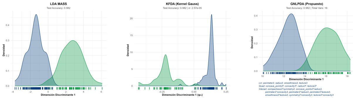
Figura 5.8: Comparativa geométrica de los espacios de proyección para el conjunto de datos Cancer Wisconsin.
