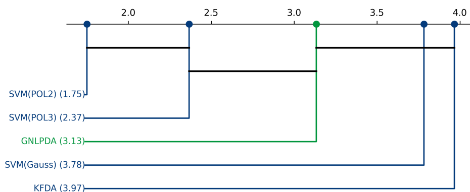
Figura 5.26: Análisis de significancia estadística post-hoc y corrección por enmascaramiento mediante distancias críticas de Nemenyi para el conjunto de datos Cancer Wisconsin.
