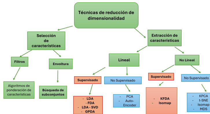
Figura 2.1: Taxonomía de las técnicas de reducción de dimensionalidad. Tomada de [43].
