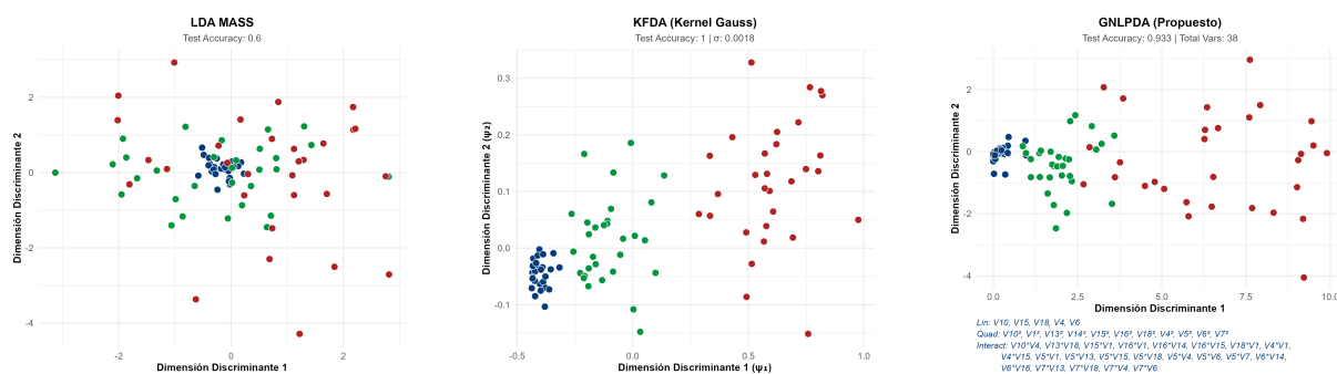
Figura 5.12: Comparativa geométrica de los espacios de proyección para el conjunto de datos cebolla 20D.
