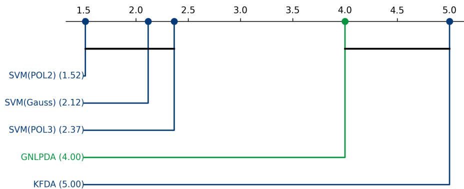
Figura 5.44: Análisis de significancia estadística post-hoc y corrección por enmascaramiento mediante distancias críticas de Nemenyi para el conjunto de datos Indicadores 2015.
