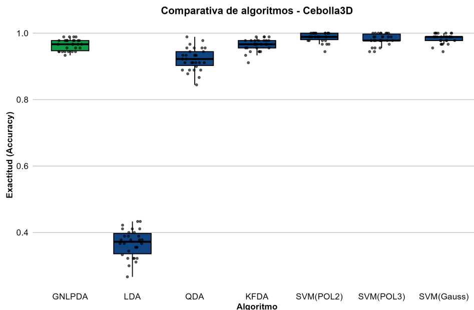
Figura 5.30: Distribución empírica del rendimiento predictivo para el conjunto de datos cebolla 3D.
