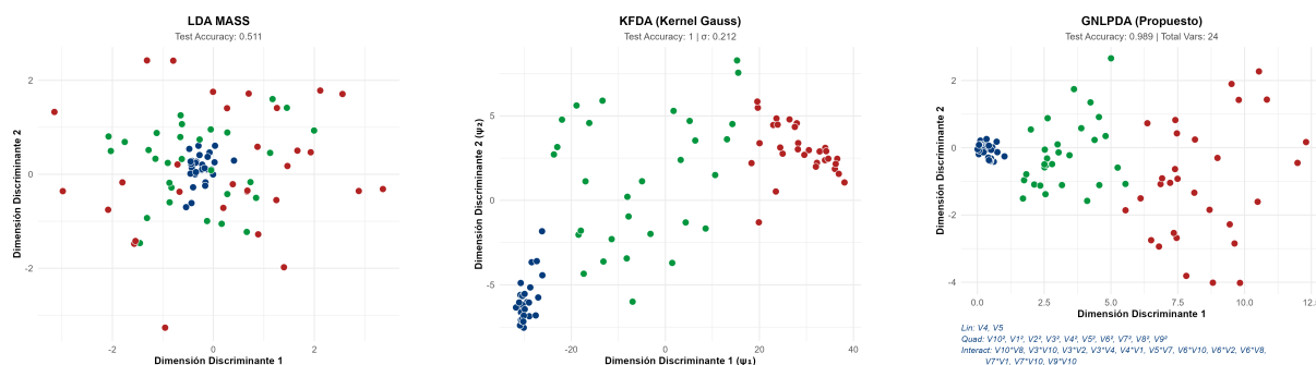
Figura 5.11: Comparativa geométrica de los espacios de proyección para el conjunto de datos cebolla 10D.
