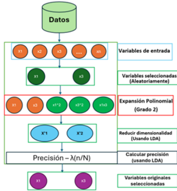
Figura 4.1: Fase I de GNLPDA: selección evolutiva de variables originales y evaluación mediante expansión polinomial y LDA. Fuente: Elaboración propia
