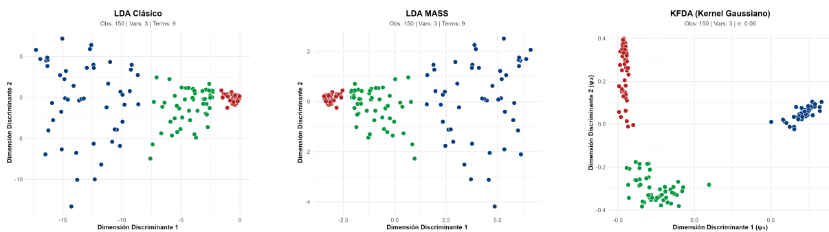
Figura 5.1: Comparativa de los espacios latentes generados por LDA, LDA MASS y KFDA ante el impacto de la alta dimensionalidad (caso 1).
