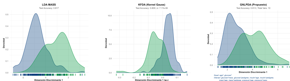
Figura 5.13: Comparativa geométrica de los espacios de proyección para el conjunto de datos Pima diabetes.
