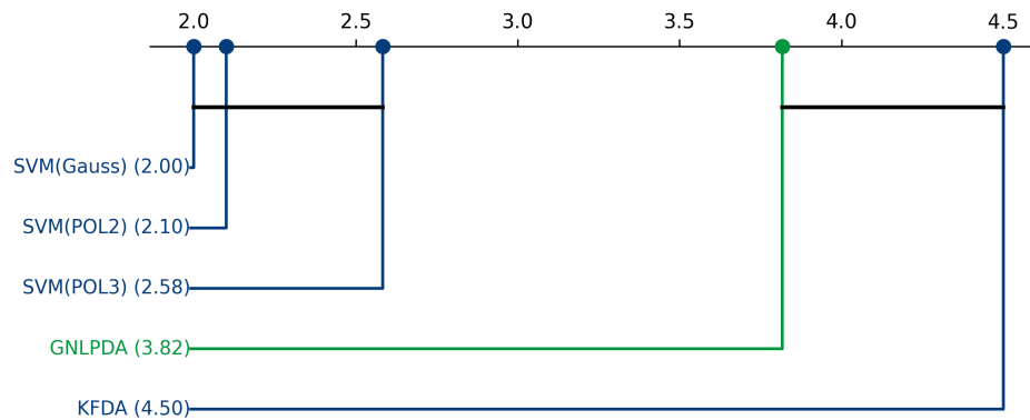
Figura 5.23: Análisis de significancia estadística post-hoc y corrección por enmascaramiento mediante distancias críticas de Nemenyi para el conjunto de datos Wines.
