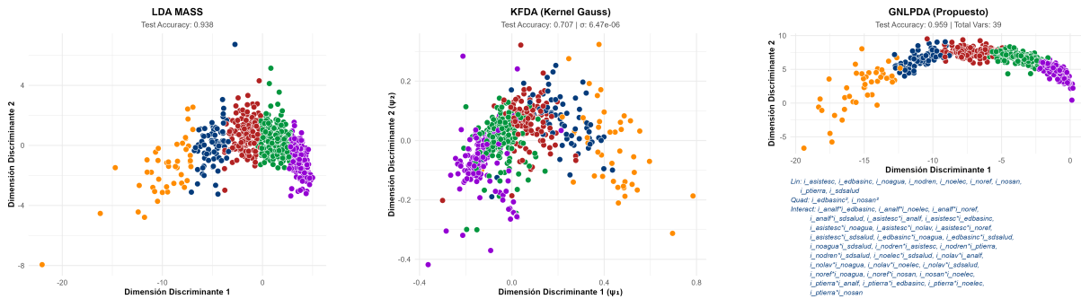
Figura 5.16: Comparativa geométrica de los espacios de proyección para el conjunto de datos Indicadores 2020 (2D).
