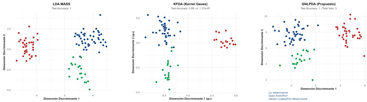
Figura 5.6: Comparativa geométrica de los espacios de proyección para el conjunto de datos Palmer Penguins.
