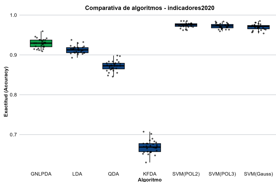
Figura 5.45: Distribución empírica del rendimiento predictivo para el conjunto de datos Indicadores 2020.
