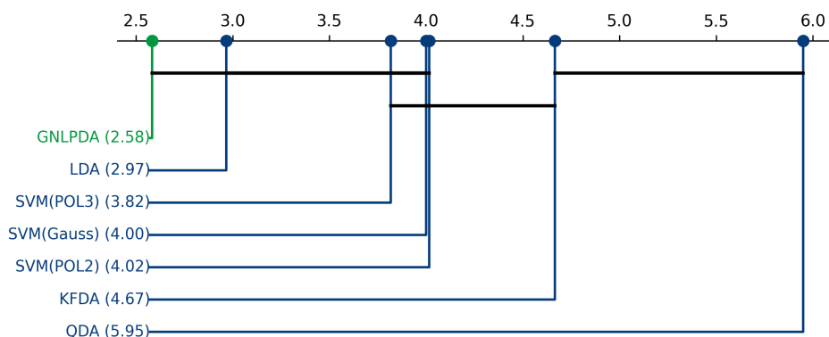
Figura 5.40: Análisis de significancia estadística post-hoc mediante distancias críticas de Nemenyi para el conjunto de datos pima diabetes.
