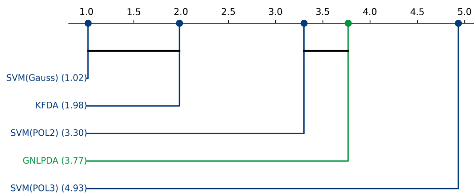
Figura 5.38: Análisis de significancia estadística post-hoc y corrección por enmascaramiento mediante distancias críticas de Nemenyi para el conjunto de datos cebolla 20D.
