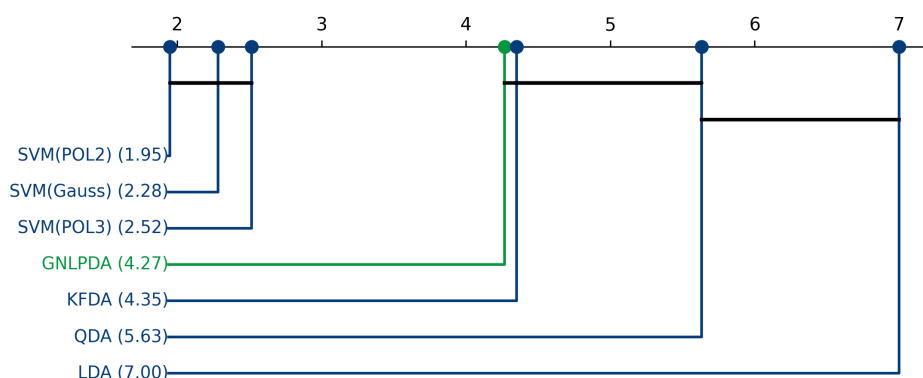
Figura 5.31: Análisis de significancia estadística post-hoc mediante distancias críticas de Nemenyi para el conjunto de datos cebolla 3D.
